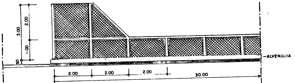
ALAMDRADO DAS QUADRAS - DETALHE - 1:100
